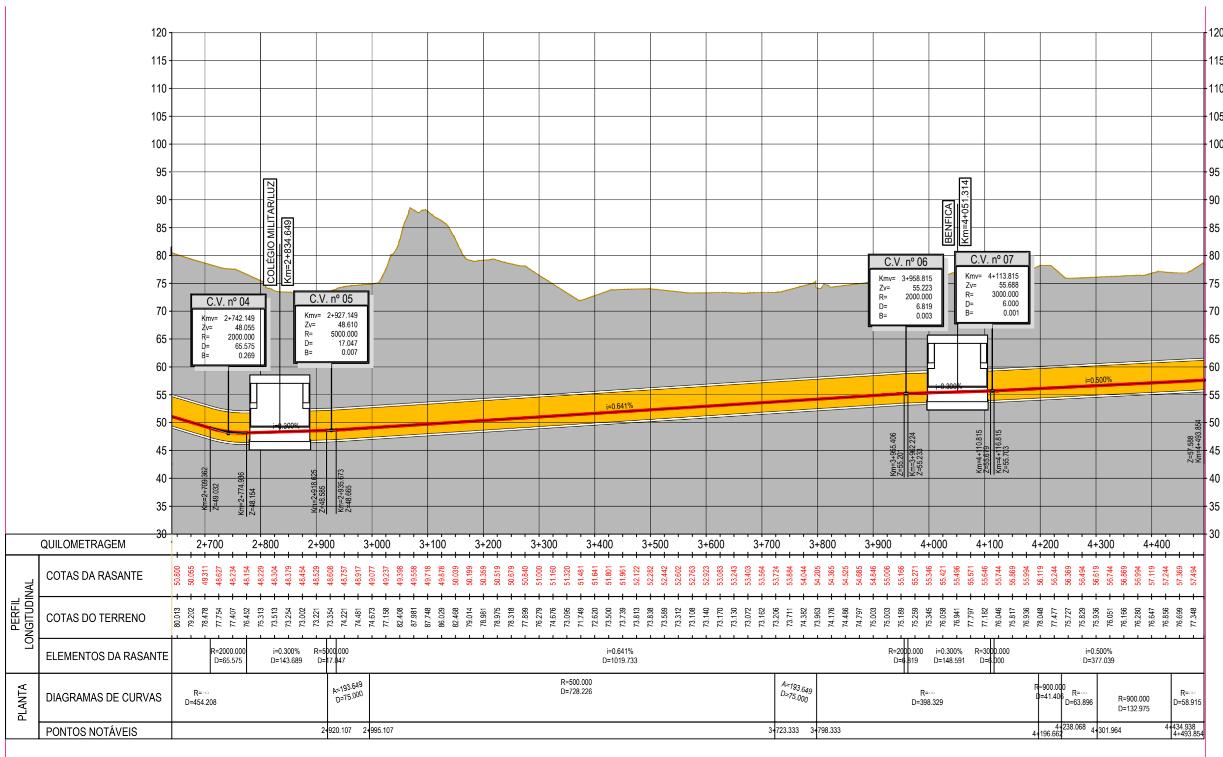
PERFIL LONGITUDINAL (Hipótese 5 e ramal de acesso ao PMO III)
